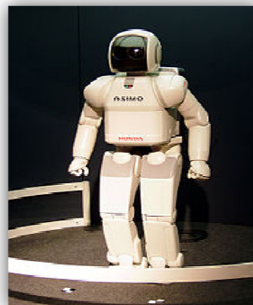
Робот-гуманоїд «Honda»
