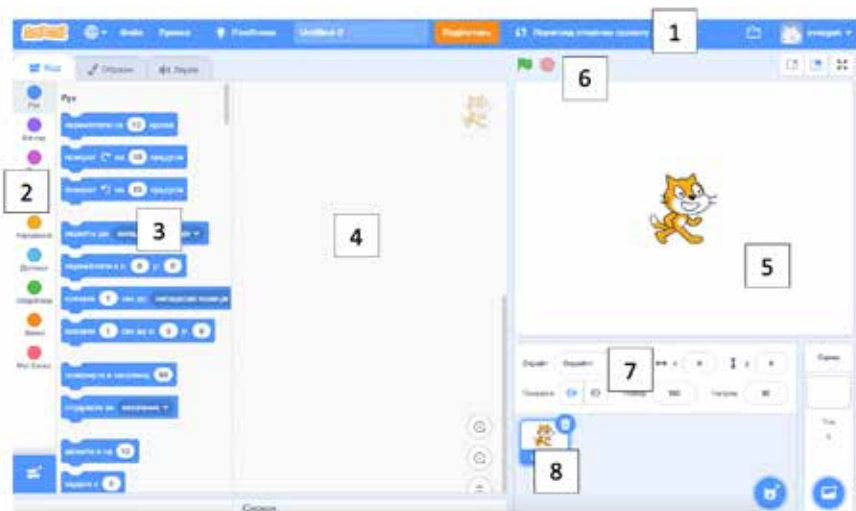
Рис. 62. Зони середовища Скретч
